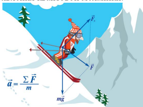
Рисунок 1 - Пример на второй закон Ньютона
